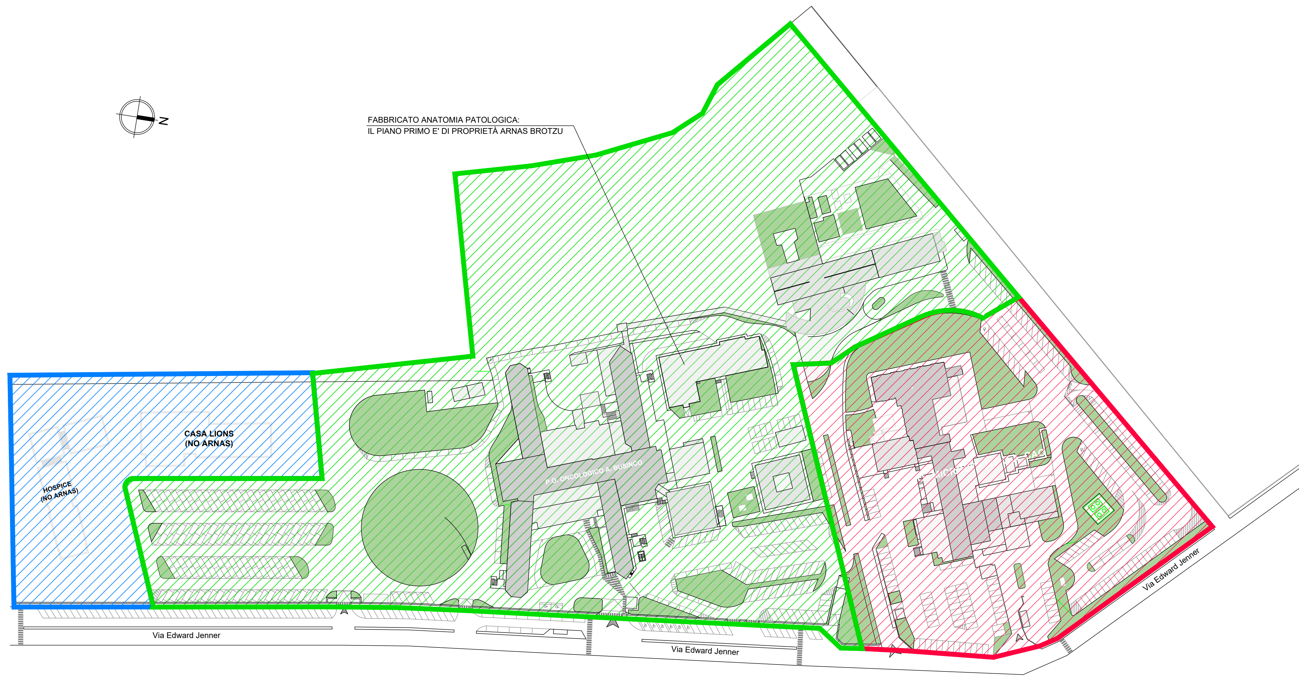
PLANIMETRIA GENERALE 1:1.000
