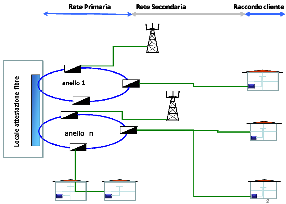
Modello architetturale
